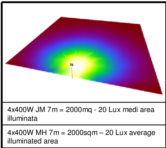
4 unità collegabili in serie con un'unica fonte di energia 4 units linkable in series with only one power source
